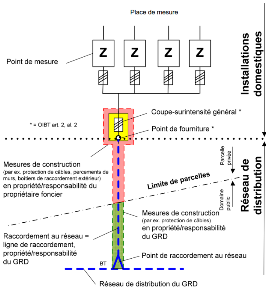
Illustration 3 : Représentation du raccordement au réseau, source : bulletin.ch 10 / 2017, article d'Olivier Stössel
